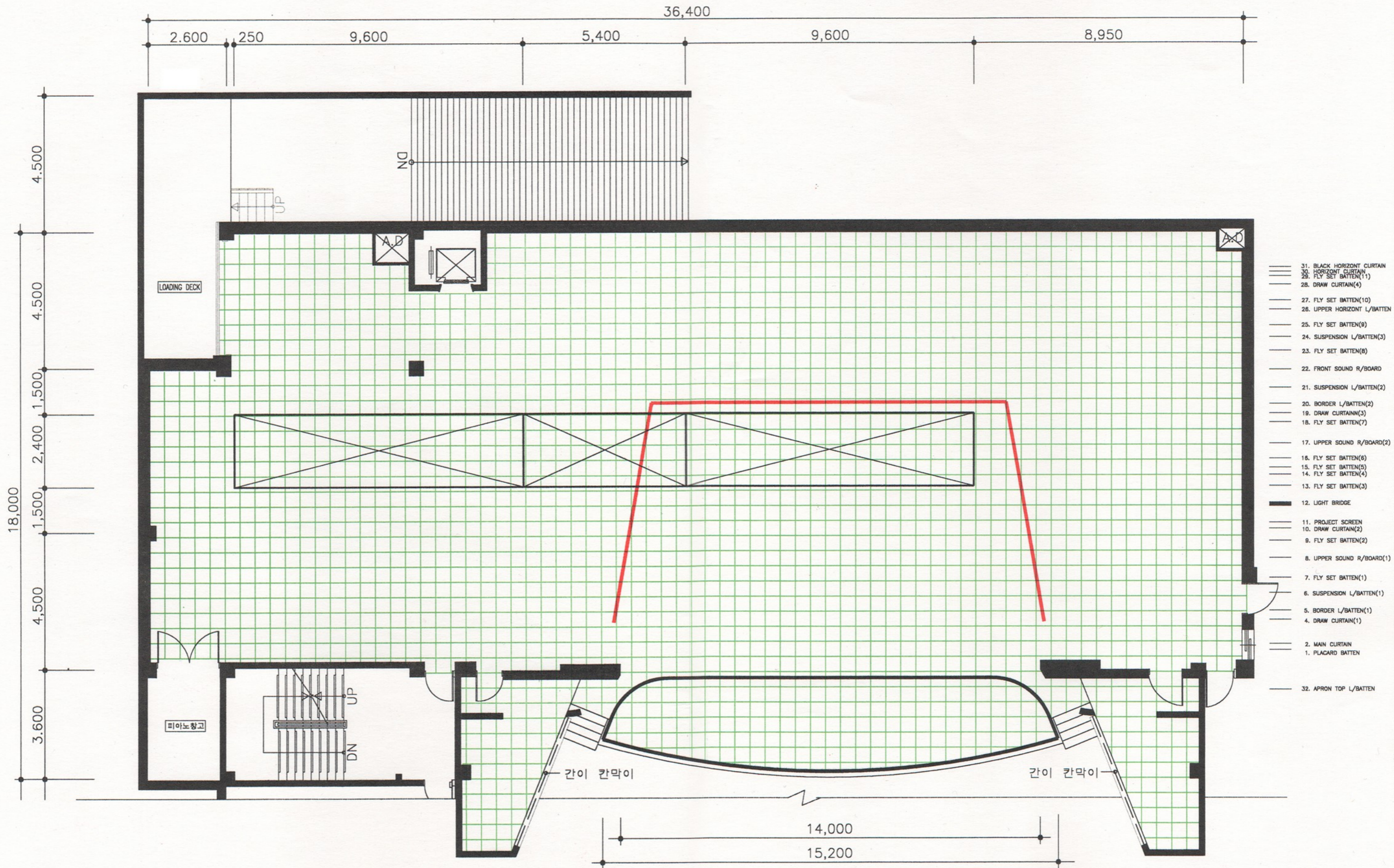
금정문화회관 대공연장 무대기기 배치도 S= 1 / 120
